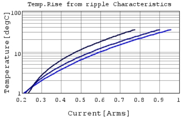
GRM1555C1H8R0CA01 Temp.rise 700MHz
